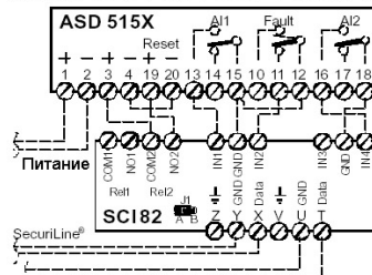
Рис. 5 SCI 82 на ASD 515-1 / ASD 515-2
