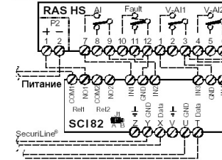
Рис. 8 SCI 82 на RAS HS
