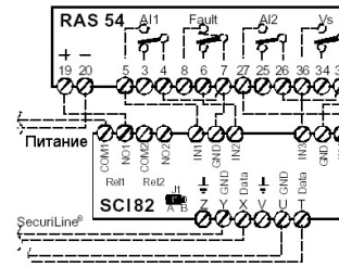
Рис. 7 SCI 82 на RAS 54
