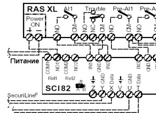
Рис. 9 SCI 82 на RAS XL
