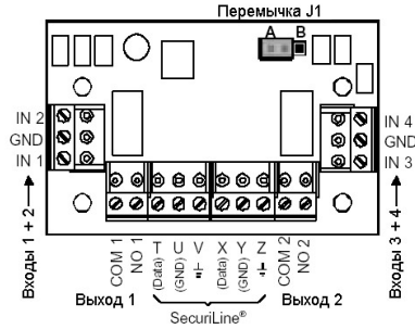
Рис. 3 Точки подключения, назначение терминала
