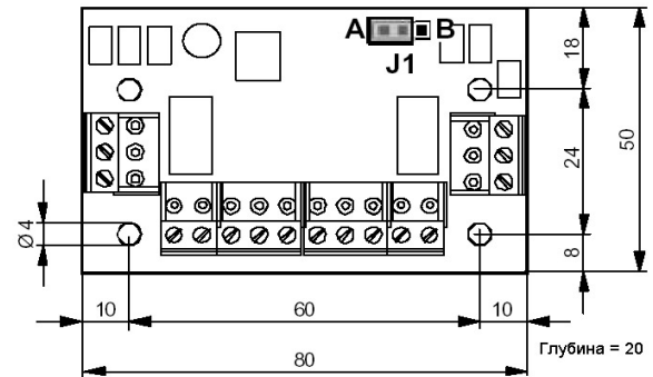
Рис. 2 Габариты SCI 82
