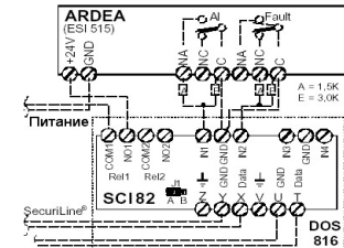
Рис. 10 SCI 82 на ARDEA ESD 515
