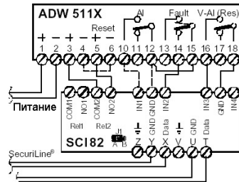
Рис. 4 SCI 82 на ADW 511 / ADW 511A / ADW 511-1
