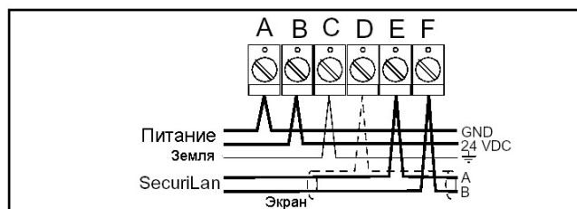
Рис. 4 Подключение PIM 731
